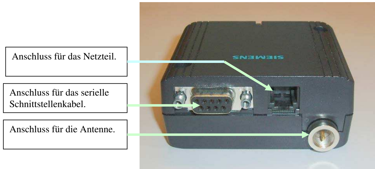
Abb. 5. GSM-Modem.
